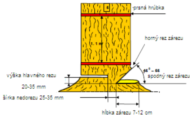
Obr. 9 - Meranie parametrov pňa
