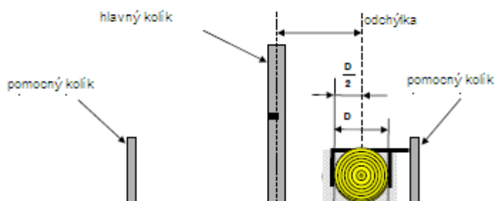
Obr. 11 - Meranie odchýlky presnosti ťažby
