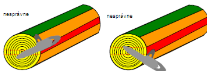
Obr. 28 - Prepílenie červenej zóny vo vnútri kmeňa
