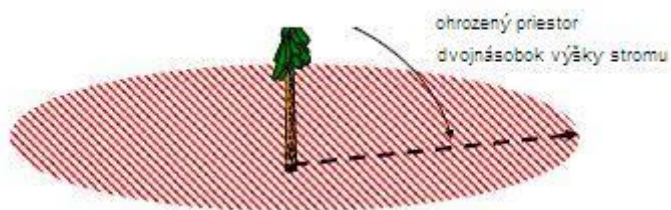
obr. 4. Ohrozený priestor pri ťažbe
