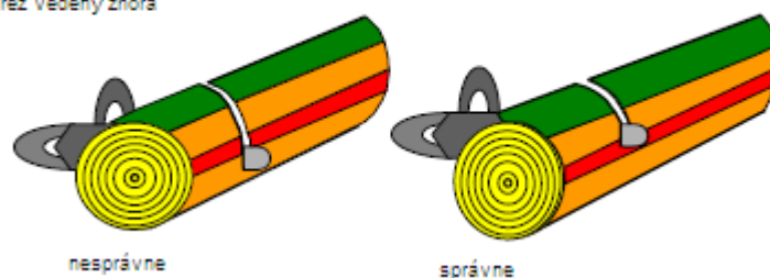
Obr. 27 - Prepílenie červenej zóny pri hornom reze rez vedený zhora
