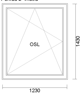
6) OKNO 1-K.(OSL) 1230x1430 Pohľad z vnútra
