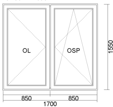
10) OKNO 2-K. (O+OS) 1700x1550 Pohľad z vnútra
