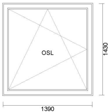
7) OKNO 1-K.(OSL) 1390x1430 Pohľad z vnútra
