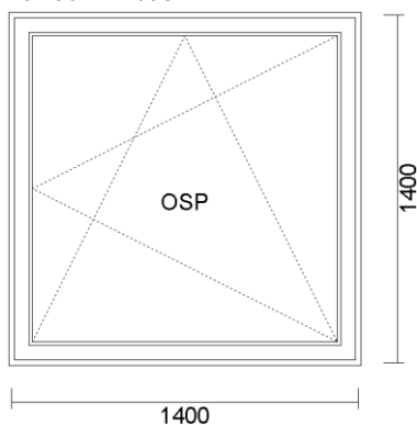
11) OKNO 1-K.(OSP) 1400x1400 Pohľad z vnútra
