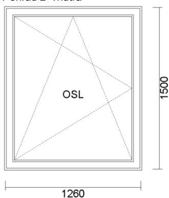
8) OKNO 1-K.(OSL) 1260x1500 Pohľad z vnútra
