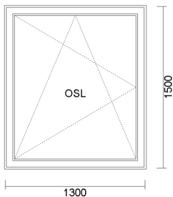
9) OKNO 1-K.(OSL) 1300x1500 Pohľad z vnútra
