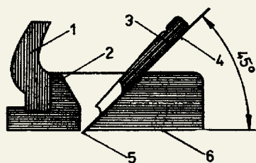
1 - kolík, 2 - lôžko, 3 - klin, 4 - železko, 5 - ústie, 6 - plaz
